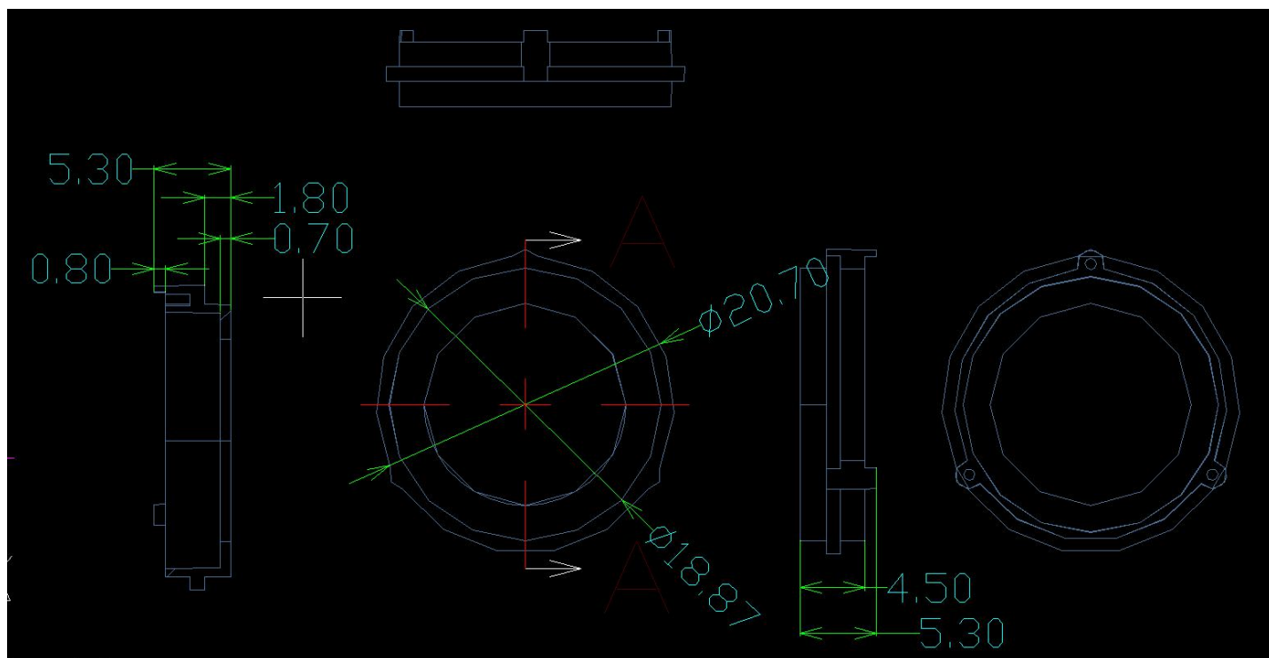
图2-1 A21尺寸图
