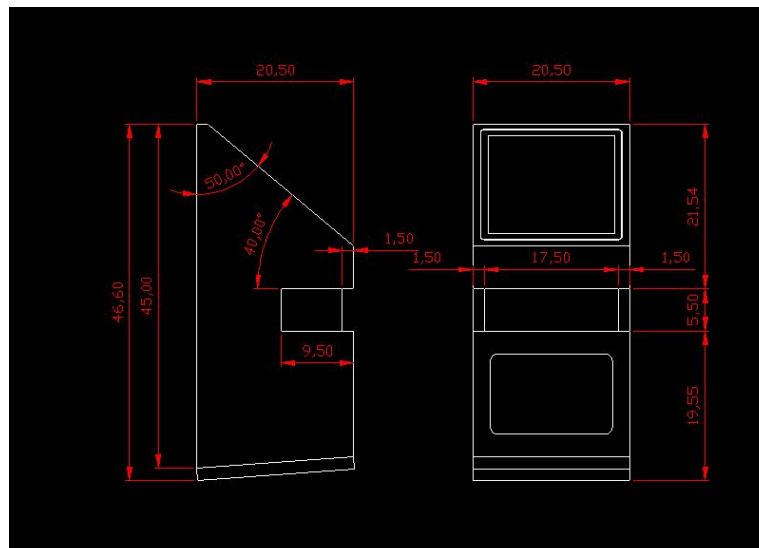
图2-1 A33尺寸图
